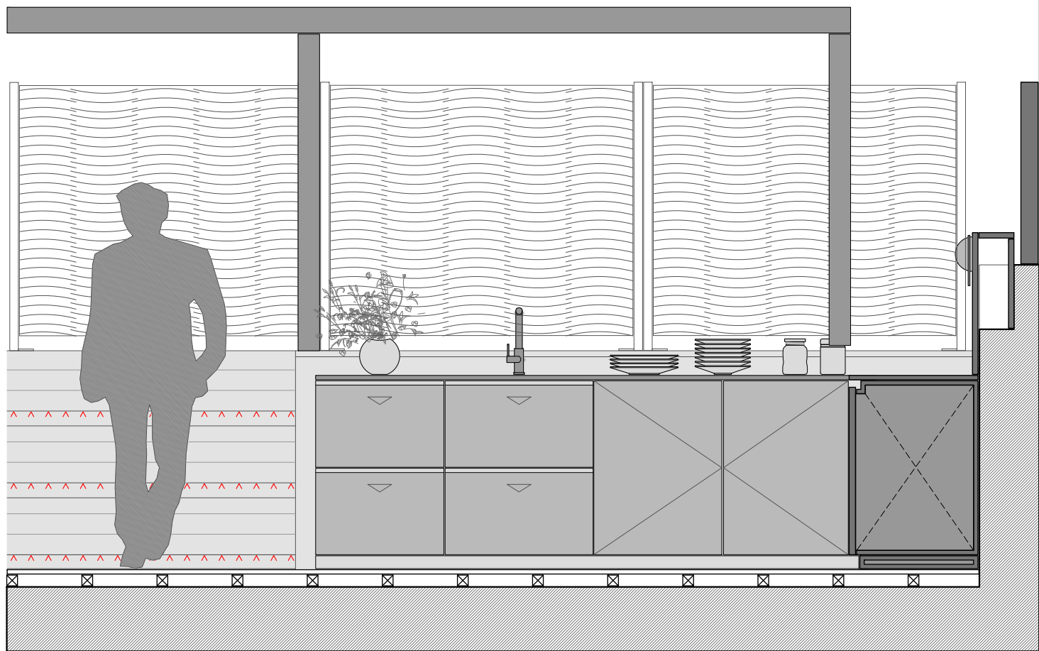
Sección E-E'
