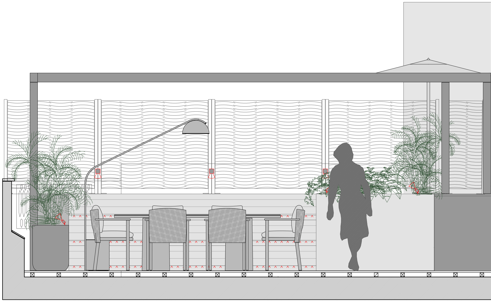
Sección C-C'
